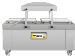
EVD-22 ■ 2 × cambra 640 × 615 × 195 mm 2 barres de 520 mm per campana Bomba 100 m³/h
