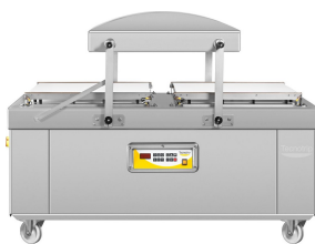
EVD-16 ■ 2 × cambra 820 × 825 × 225 mm 2 barres de 720 mm per campana Bomba 150 o 250 m³/h
