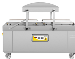
EVD-19 ■ 2 × cambra 955 × 895 × 250 mm 2 barres de soldar a cada campana 2 versions Opció de tapa automàtica Bomba 250 m³/h
